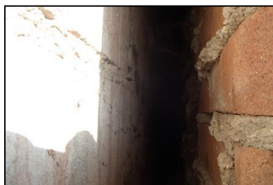
Figuur 15. Brede spouwmuur.
