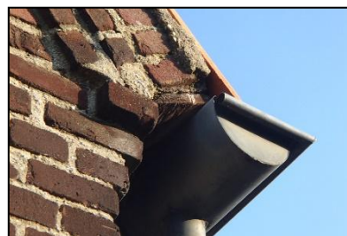
Figuur 17. Geen opening tot dakbeschot.
