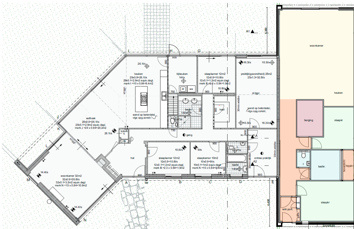
Figuur 3.1. De voorgestane situatie. Bron: mc-architecten bv.
