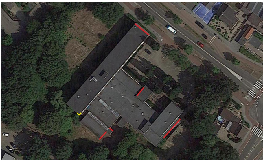
Figuur 4.4.3. Op verschillende locaties bevinden zich openingen die vleermuizen toegang kunnen geven tot de spouw. Het betreft hier voornamelijk open stootvoegen (rode lijnen) en op een plek ontbreken enkele bakstenen (gele lijn).
