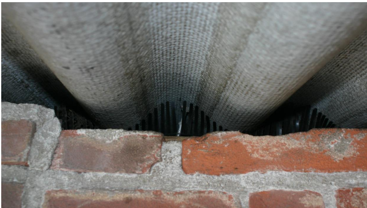
Figuur 4.2.1. Bevestigde vogelschroot tussen de muur en de golfplaten daken.
