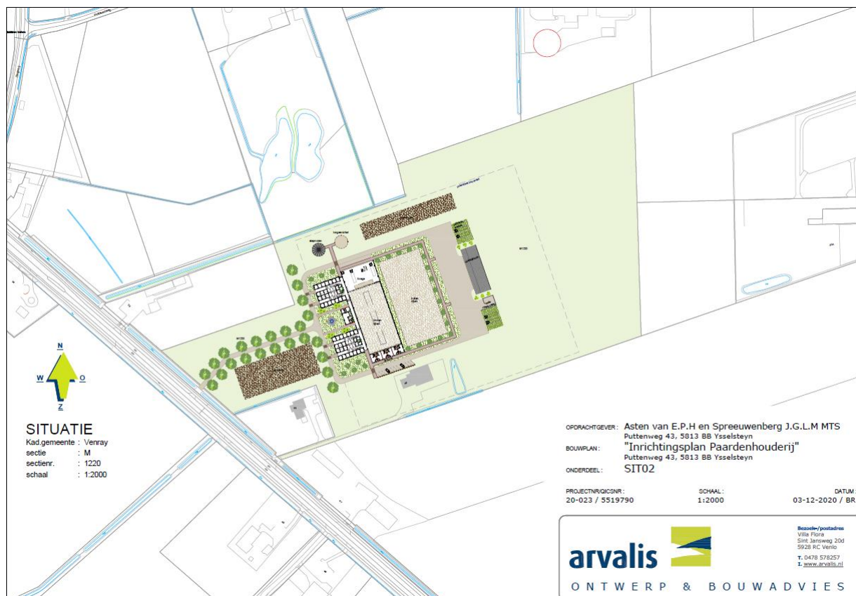
Figuur 3.1 Voorgestane situatie. Bron: Arvalis.
