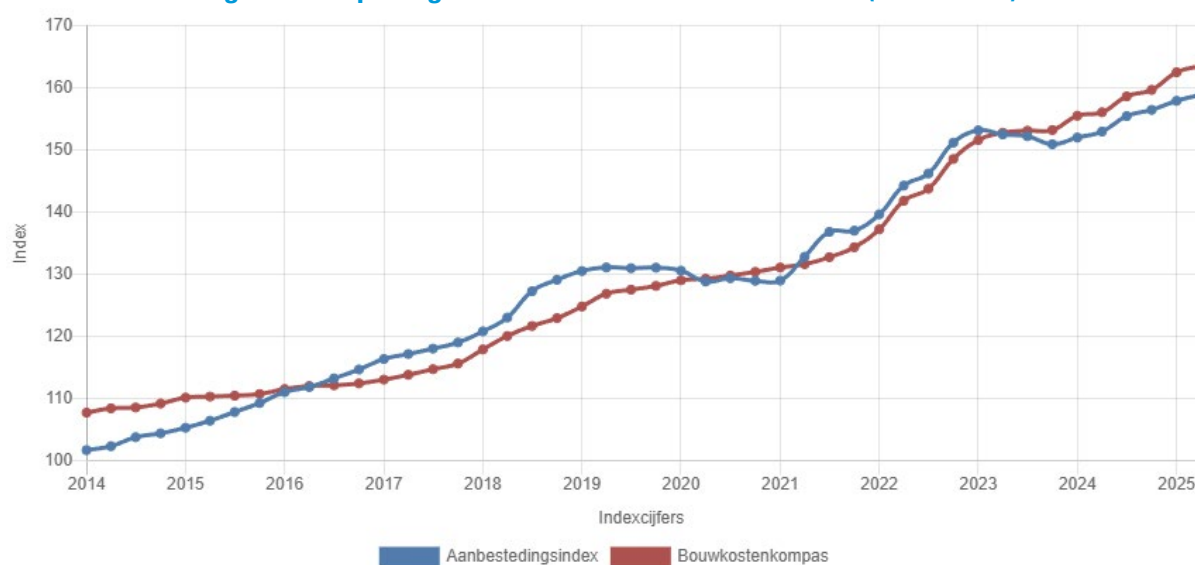
Figuur 7: Ontwikkeling en voorspelling bouwkosten voor utiliteitsbouw (2007 = 100)
